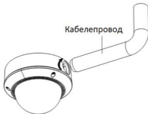
Рисунок 2-10 Установка кабелепровода
