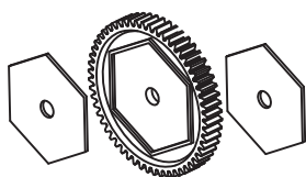
Ведомая шестерня 68Т с пластинами слиппера (E10 - XT MT)
