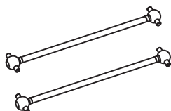
Полуось 96.4мм (E10 - XT MT)
