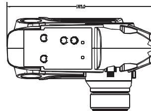
РАЗМЕРЫ ПЕРЕДАТЧИКА
