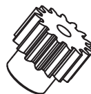
Модуль 0.8 Моторная шестерня (17Т)
