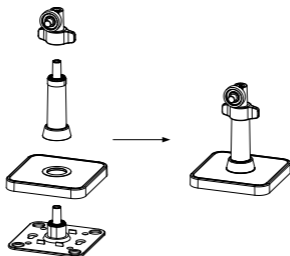
Рисунок 3-1 Сборка подставки
