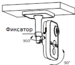
Рисунок 3-6 Регулировка камеры
