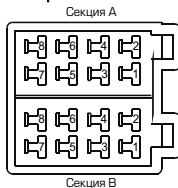
Расположения контактов разъема ISO:
