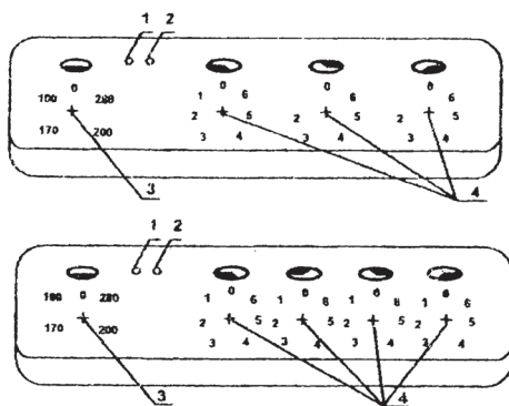
Рис. 2. Панель электроплиты (трех и четырехконфорочная) 1 – сигнализация включения жарочного шкафа; 2 – сигнализация включения электроконфорок; 3 – ручка управления жарочным шкафом; 4 – ручки управления электроконфорками.
