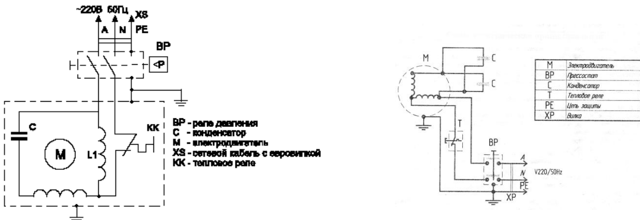
Рис. 2. Схема электрическая принципиальная
