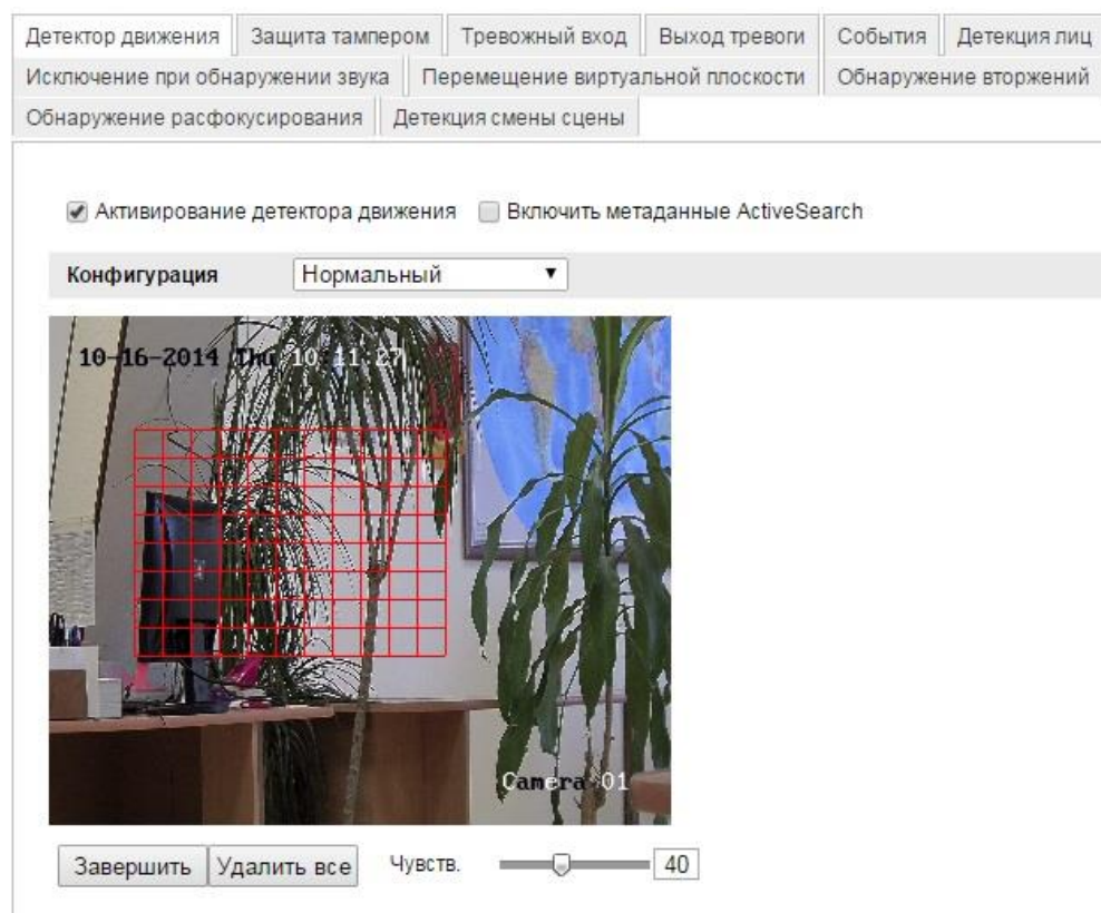
Рисунок 6-33 Настройка детектора движения
