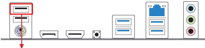
USB-BIOS-Flashback-Port
