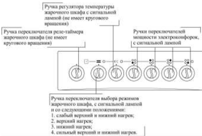
Рис. 9 Передняя панель плиты ЭПС43р1 МС
