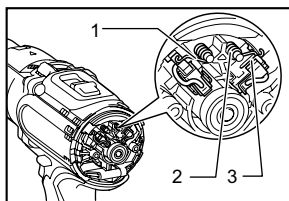
1. Brazo 2. Resorte 3. Parte rebajada
