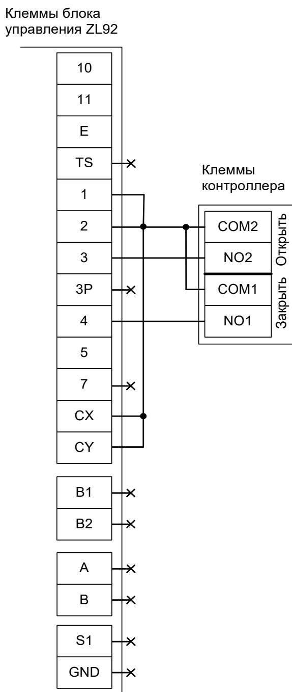
Рисунок 185. ZL92 с потенциальным управлением.
