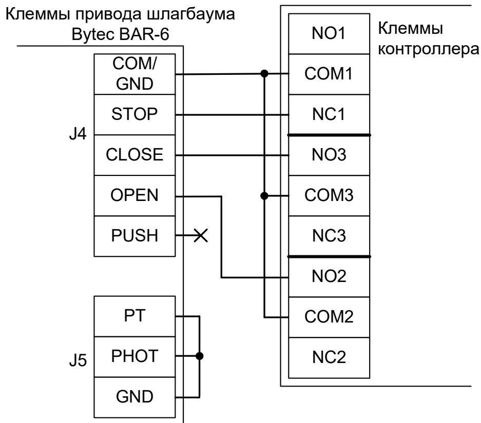
Рисунок 215. Bytac BAR-6, Skyros B-56, B-76.
