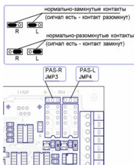
Рисунок 94. Перемычки JMP3 и JMP4 контроллера OMA 264MC1.
