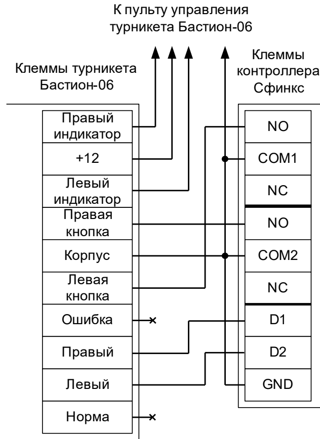
Рисунок 110. «Бастион-06» и «Бизон».
