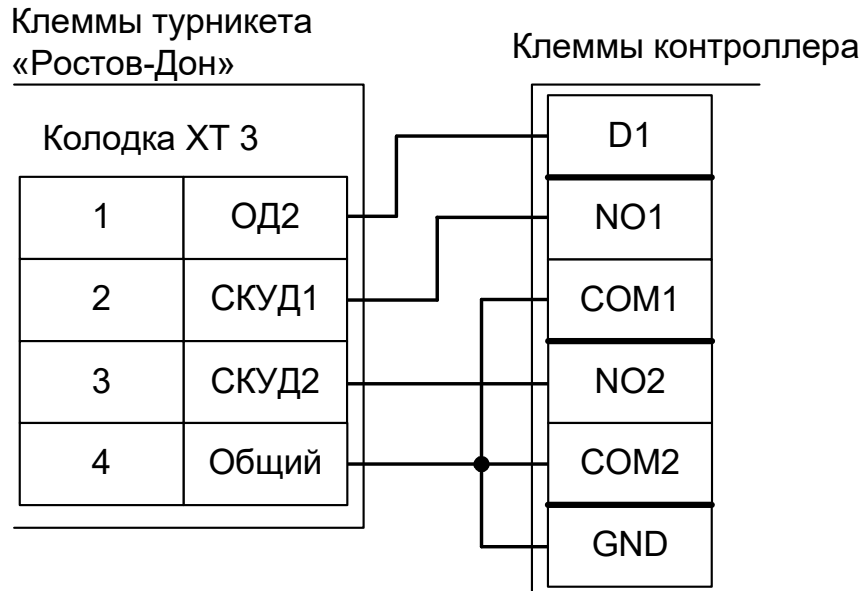
Рисунок 102. Турникеты и калитки «Ростов–Дон», старая электроника, вариант №1.
