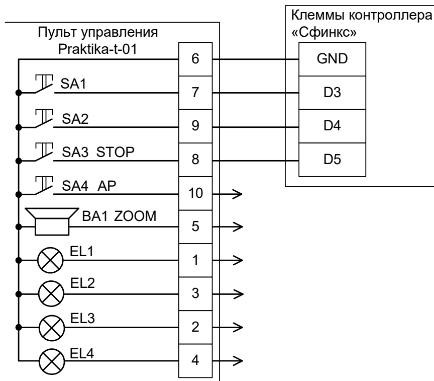
Рисунок 118. Старый пульт управления Praktika.
