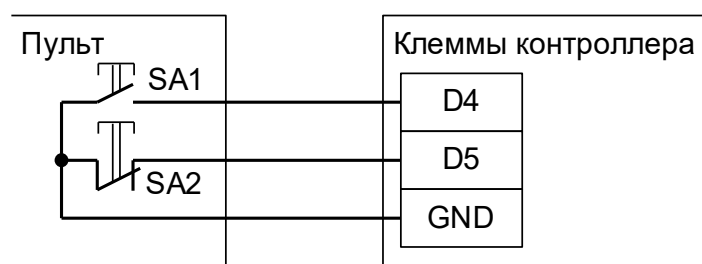
Рисунок 154. Пульт ручного управления шлагбаумом/воротами, вариант №2.
