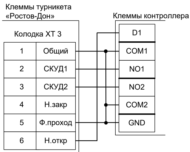
Рисунок 105. Турникеты и калитки «Ростов-Дон», старая электроника, вариант №4.
