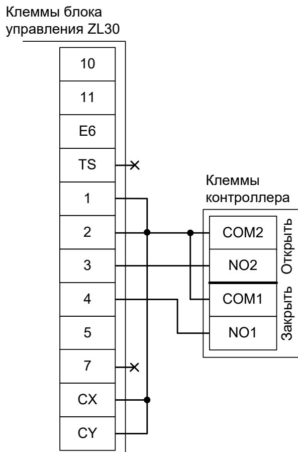
Рисунок 187. ZL30 с потенциальным управлением.
