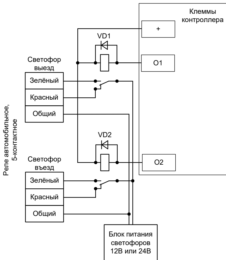
Рисунок 157. Подключение светофоров к внешним реле.
