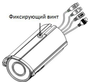
Рисунок 2-1 Удаление солнцезащитного козырька (1)
