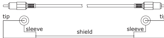
Fig. 3.5: RCA cable
