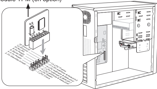
Module TPM (en option)
