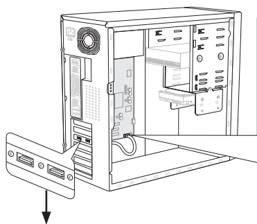
Кронштейн USB 3.0 (дополнительно)
