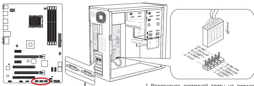
Кронштейн USB 2.0 (дополнительно)
